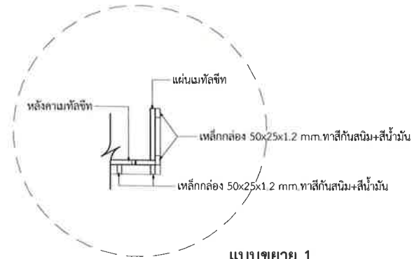
แบบขยาย 1
