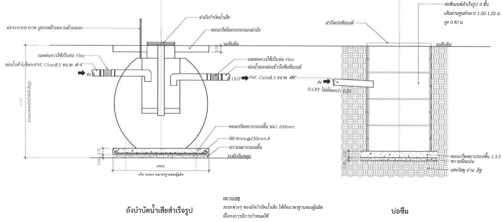
แบบขยายถังบำบัดน้ำเสียสำเร็จรูป - บ่อซึม
