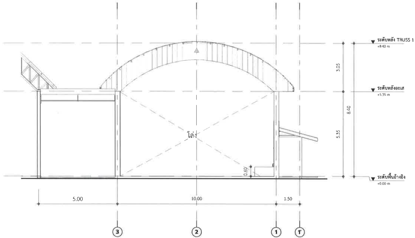
รูปด้าน 03
