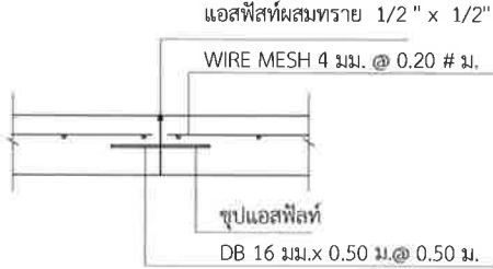
แบบขยายเทลานคอนกรีต SCALE (A3) 1 : 20
