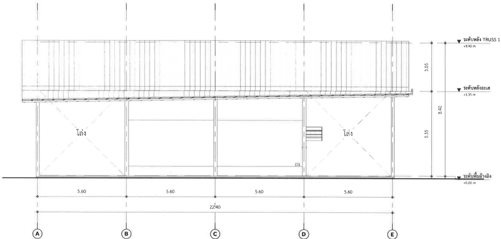
รูปด้าน 04
