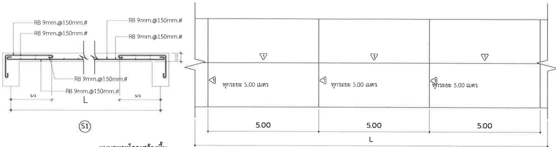
แปลนเหล็กเสริมคอนกรีต SCALE (A3) 1 : 75
