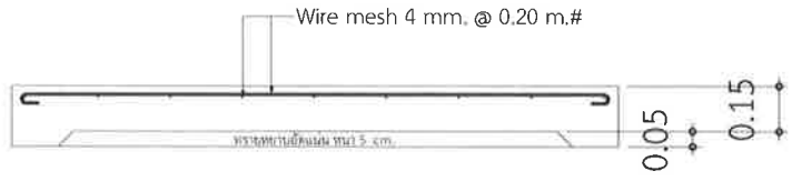
แบบขยายโครงสร้างพื้น SCALE (A3) 1 : 20
