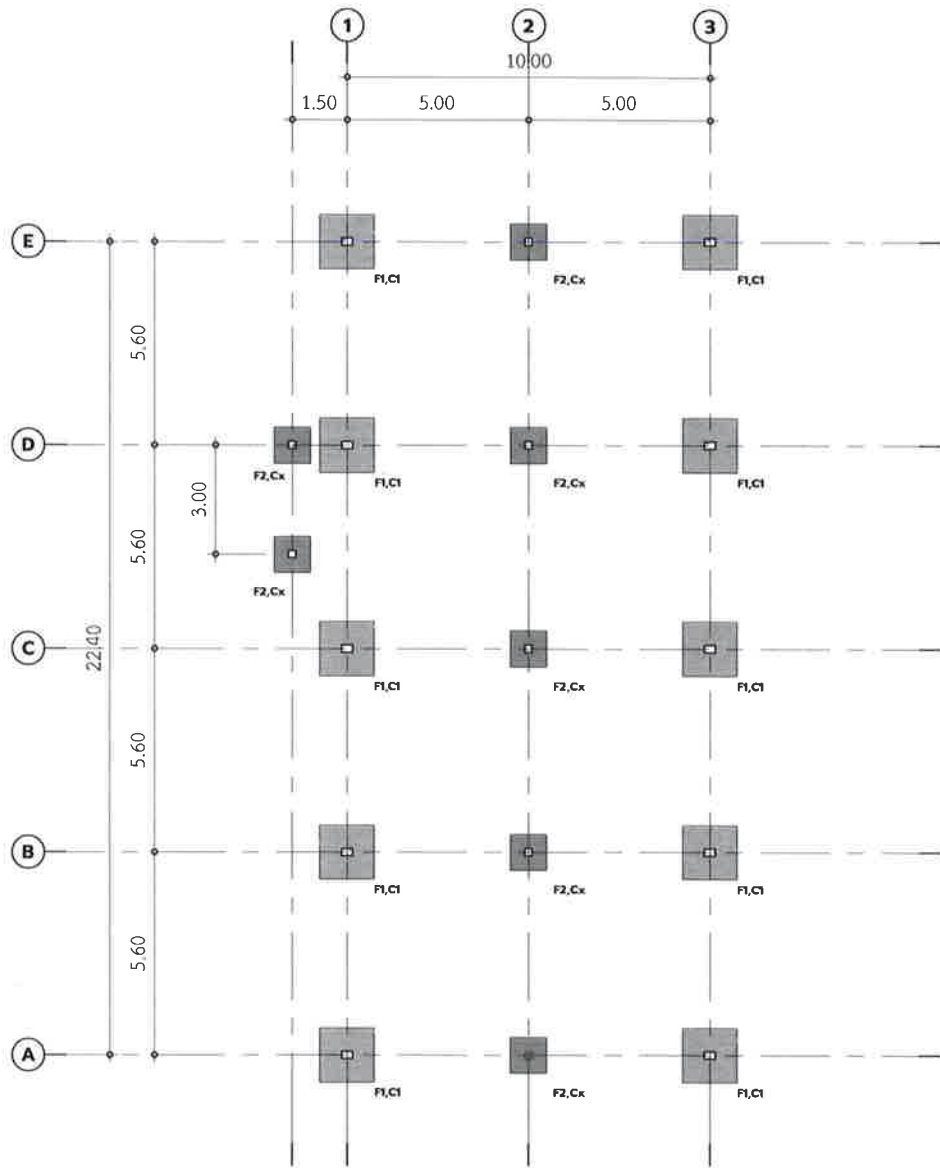
แปลนโครงสร้างฐานราก
