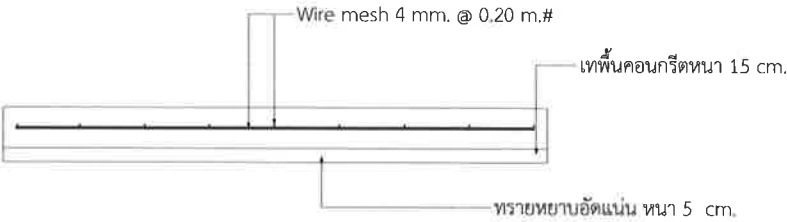
แบบขยายเทลานคอนกรีต SCALE (A3) 1 : 20
