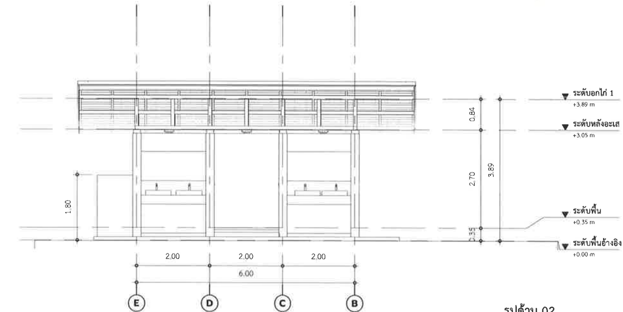
รูปด้าน 02
