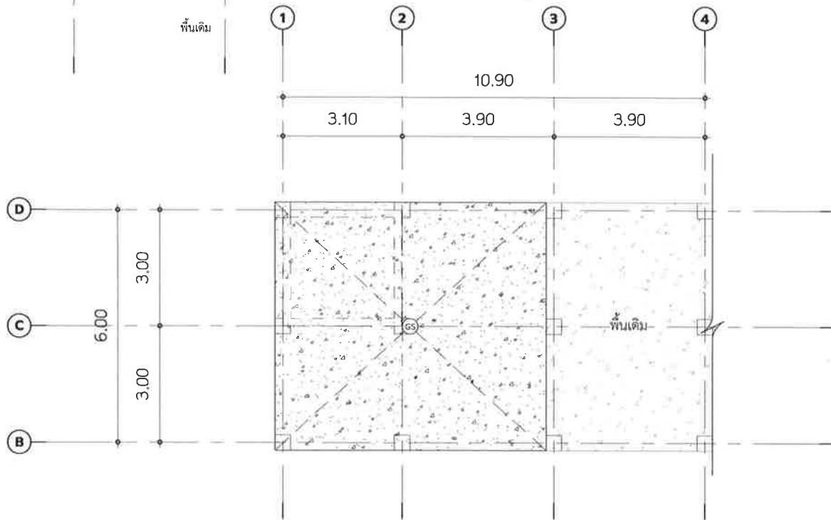
แบบขยายโครงสร้างพื้น
