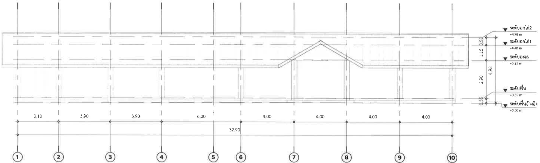
รูปด้าน 01
