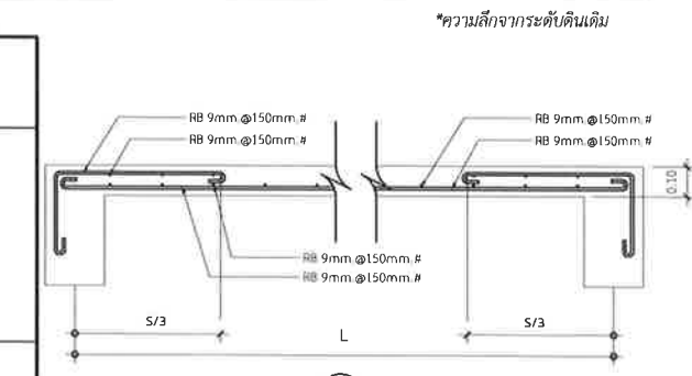
แบบขยายโครงสร้างพื้น
