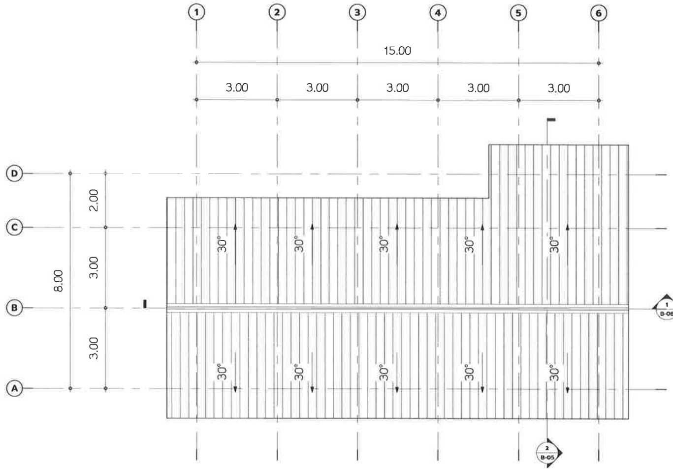
แปลนหลังคา
