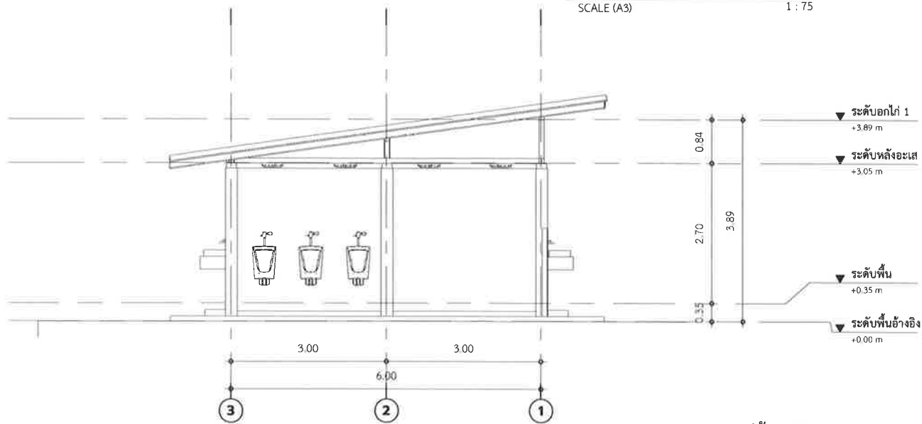
รูปด้าน 03
