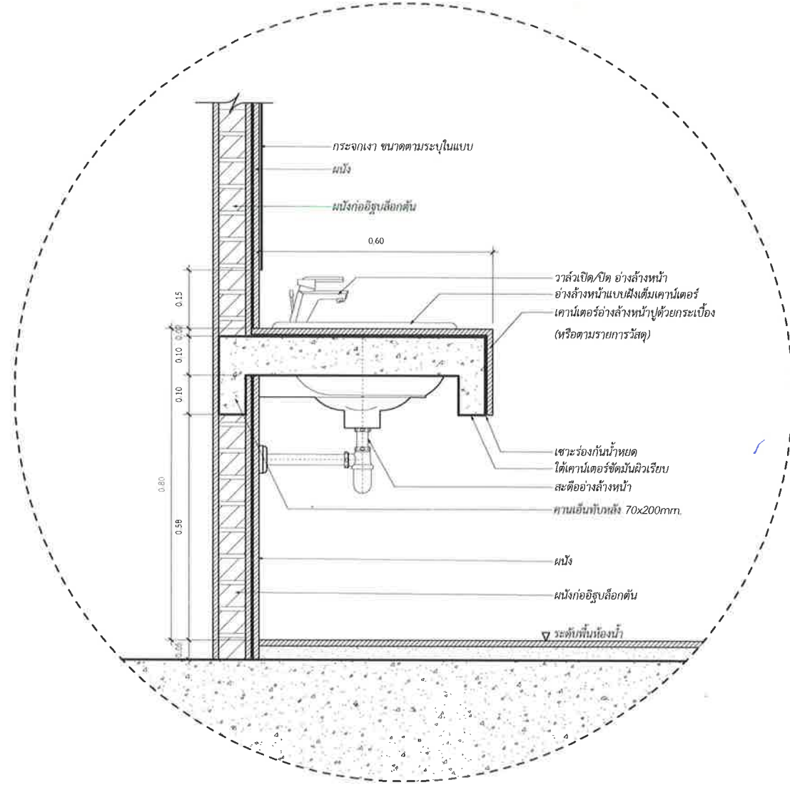
แบบขยายอ่างล้างหน้า
