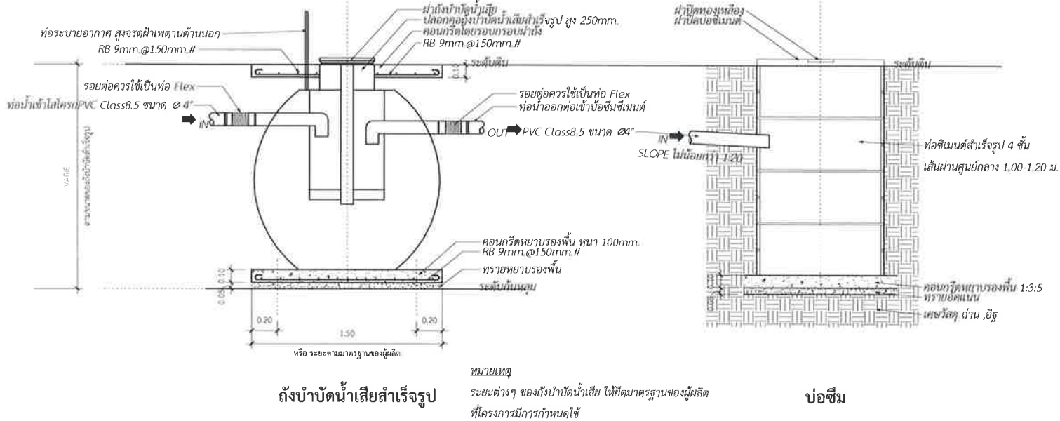
แบบขยายถังบำบัดน้ำเสียสำเร็จรูป - บ่อซีเมนต์
