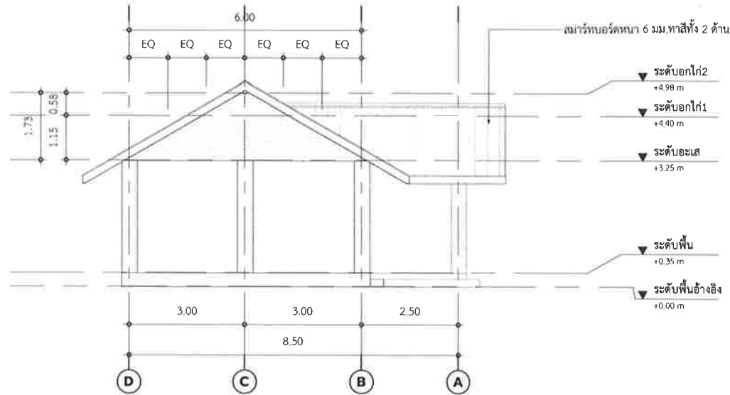
รูปด้าน 02
