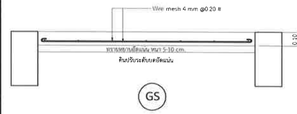
แบบขยายโครงสร้างพื้น
