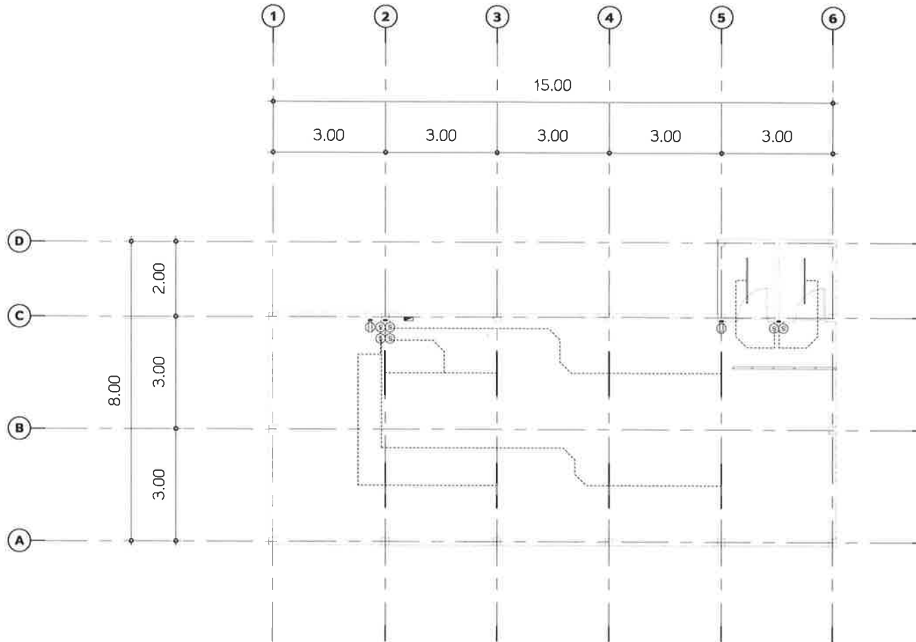
แปลนไฟฟ้ากำลังและส่องสว่าง
