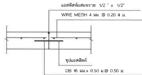
แบบขยาย CONTRACTION JOINT
