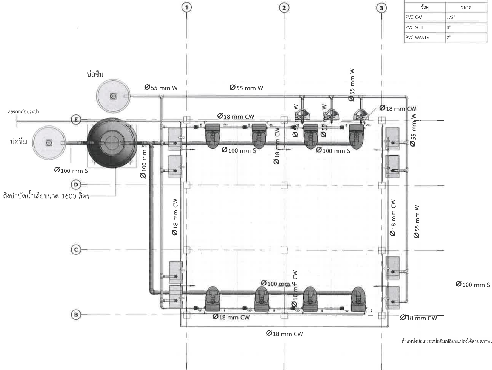
แปลนระบบประปา, สุขาภิบาล
