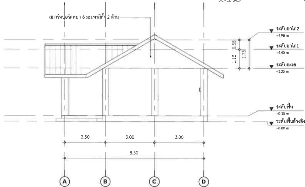
รูปด้าน 02
