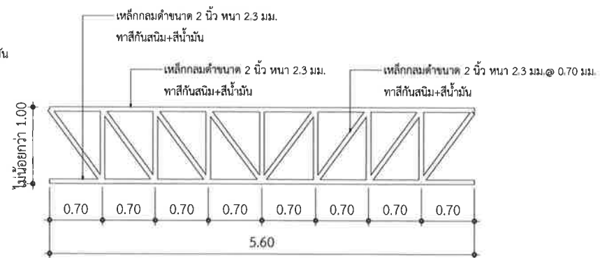
แบบขยาย T3
