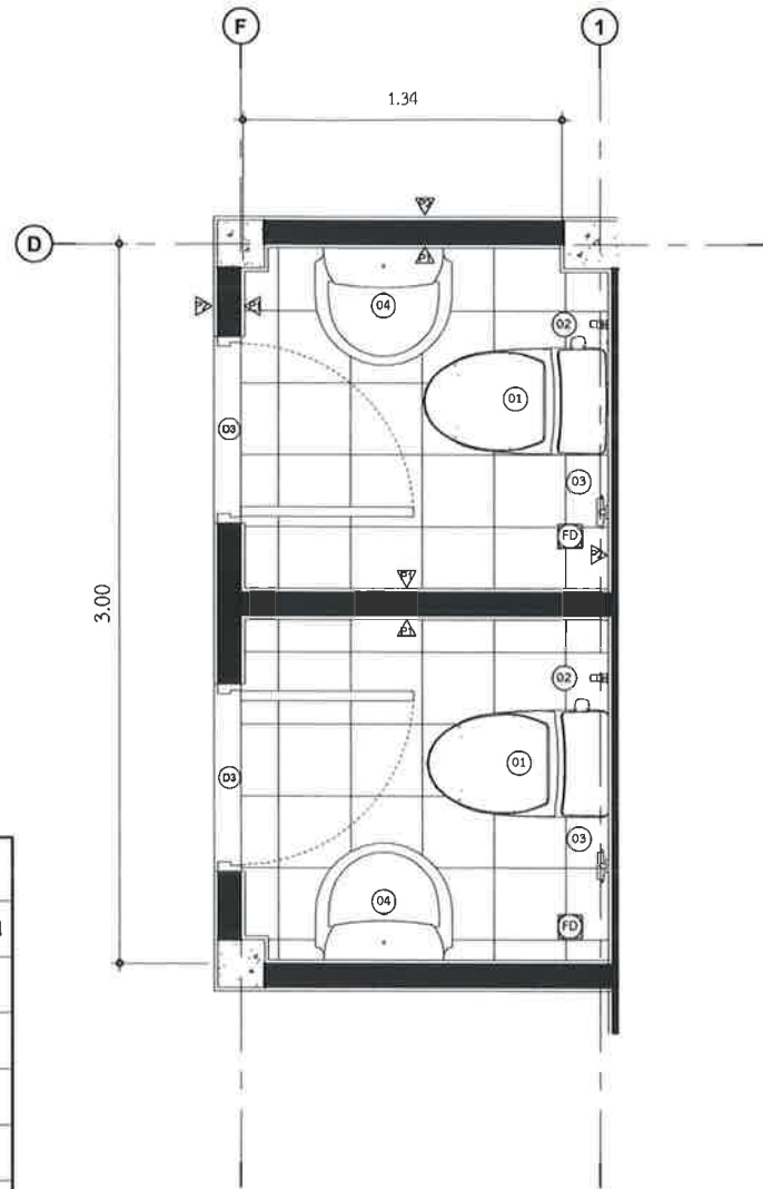
แบบขยายห้องน้ำ
