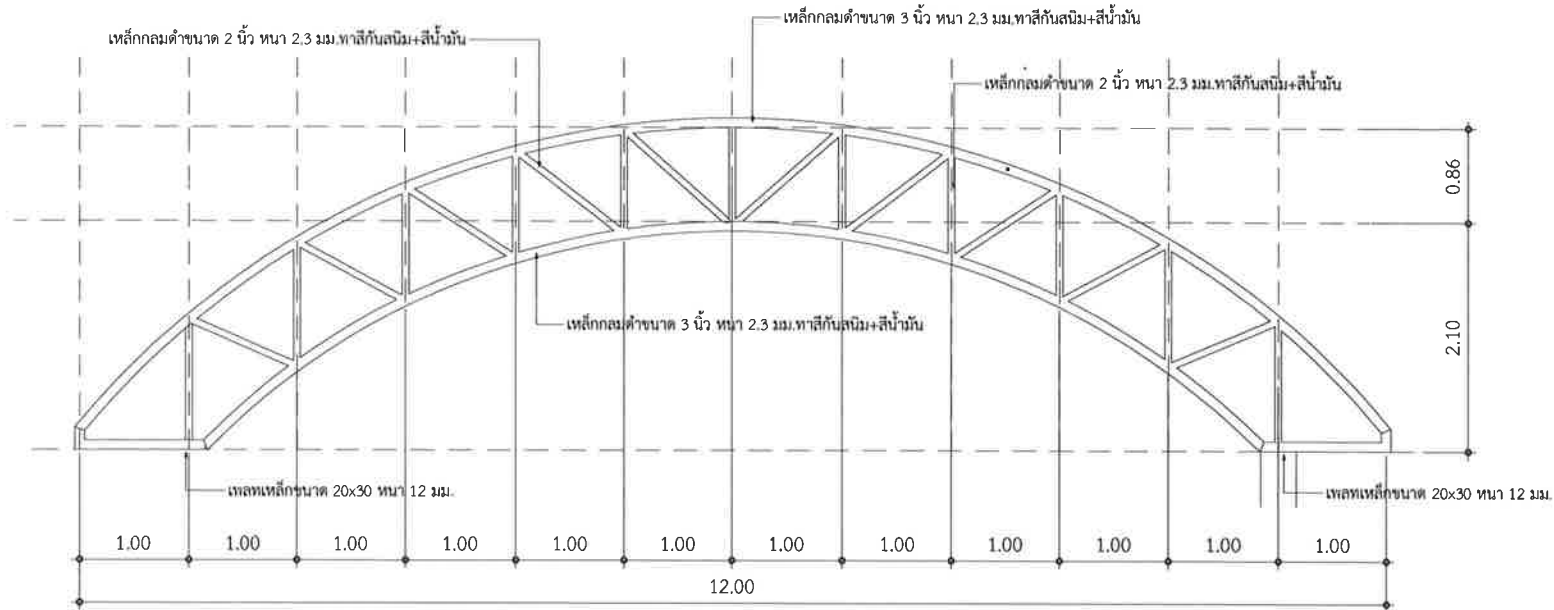
แบบขยาย T1
