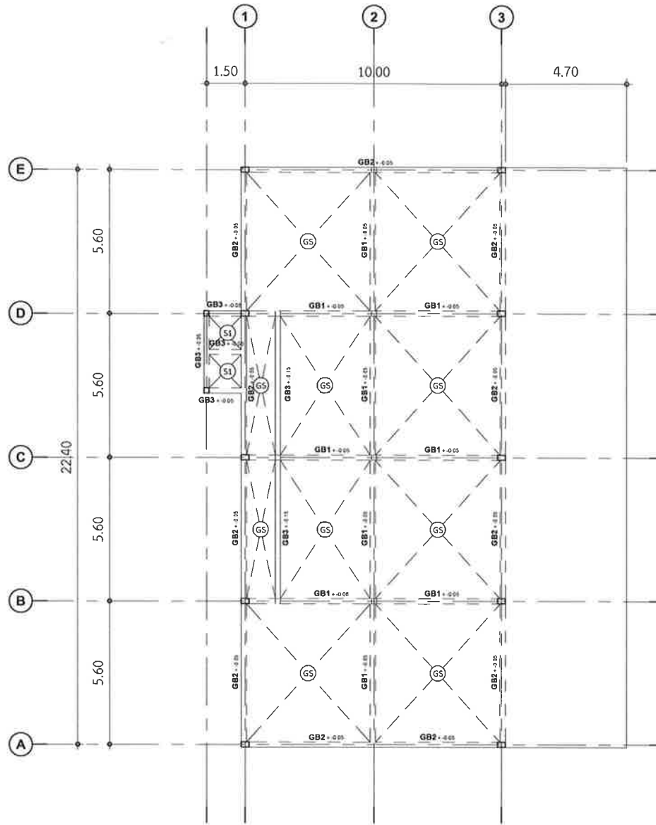
แปลนโครงสร้างคาน, พื้น
