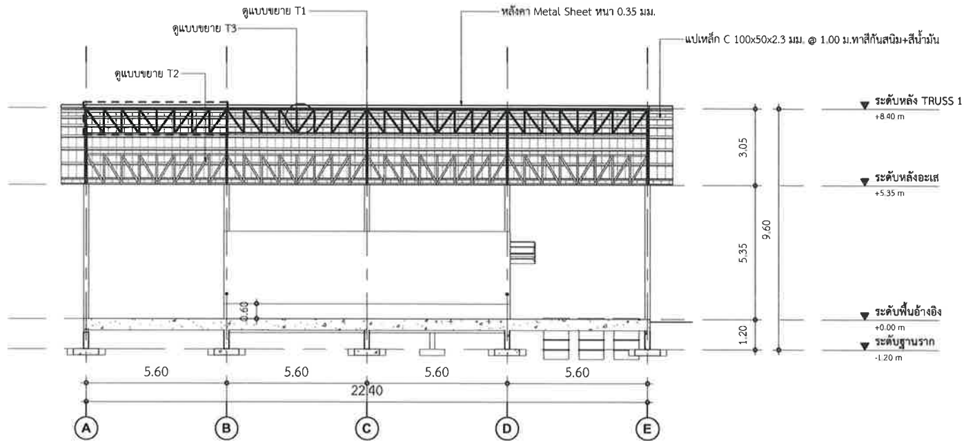
รูปตัด 02
