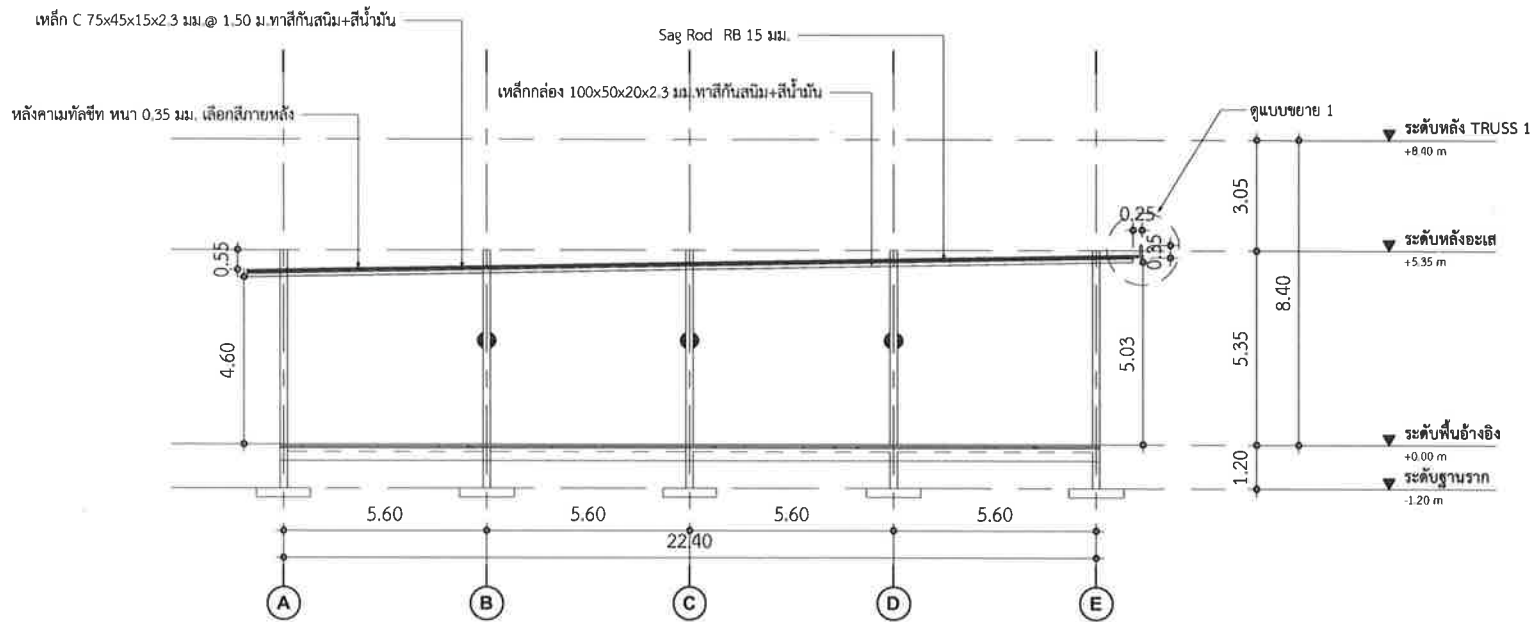
รูปตัดวางริน
