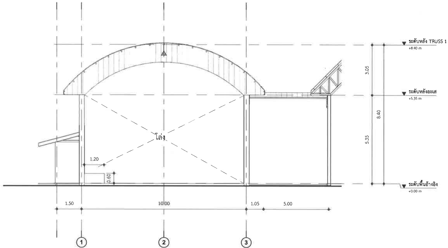
รูปด้าน 01
