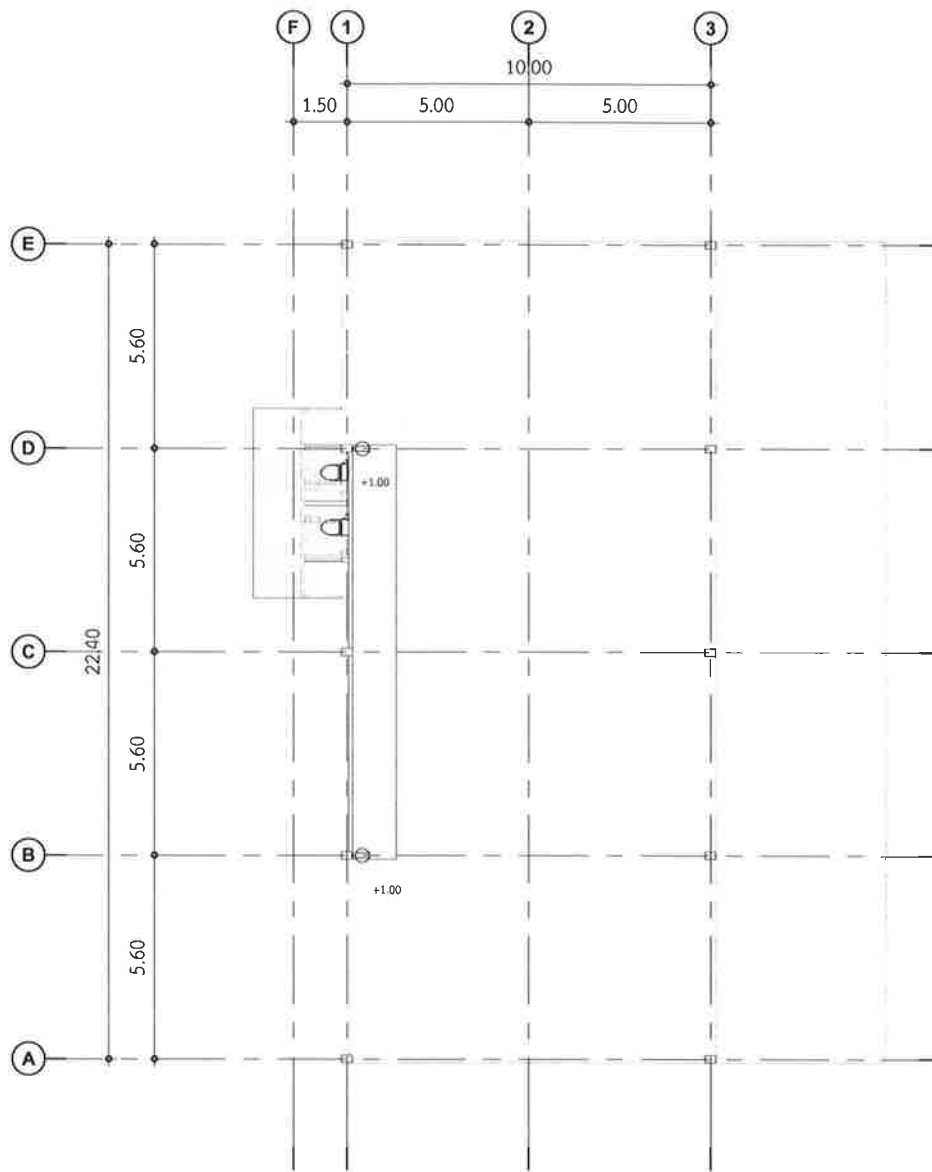
แปลนไฟฟ้ากำลัง
