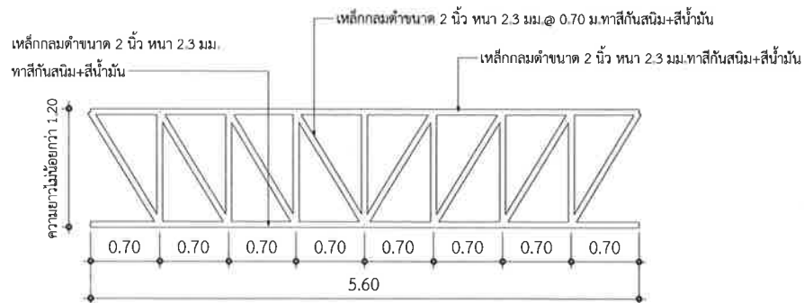
แบบขยาย T2
