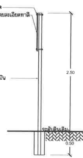
แบบรูปด้านข้างบ่อบั่โครงการ 1:25
