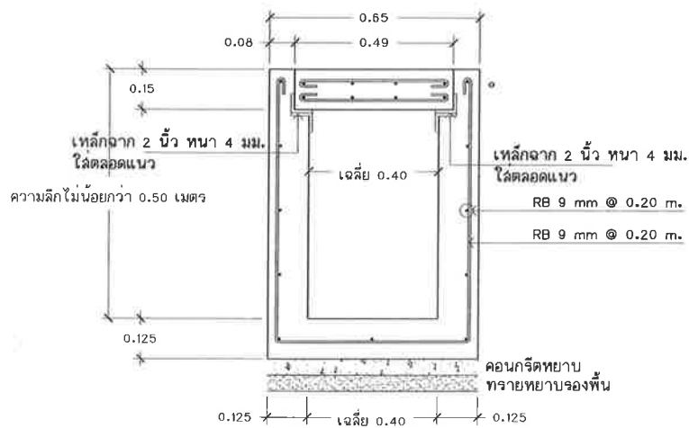
รูปตัดวางระบายน้ำ จุดที่ 1 STA 0+000 ม. Scale no
