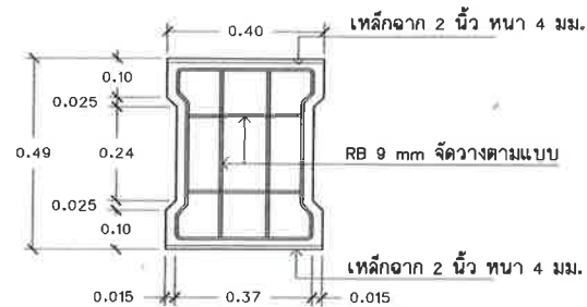
แปลนฝังวางระบายน้ำความกว้างภายในเฉลี่ย 0.40 เมตร(หรือเฉลี่ยตามสภาพพื้นที่) Scale 1:15
