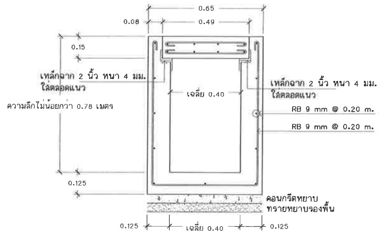
รูปตัดวางระบายน้ำ จุดที่ 1 STA 0+020 ม. Scale no
