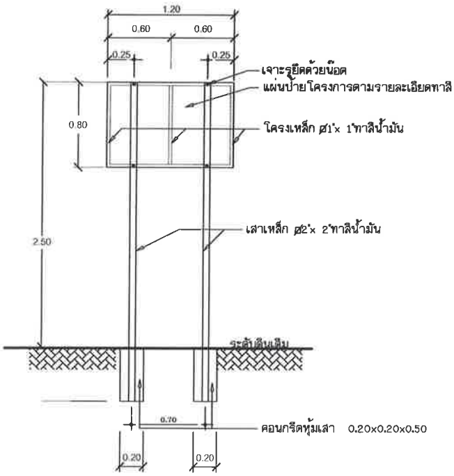
แบบรูปโครงเหล็กบ่อบั่โครงการ 1:25
