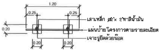
แบบรูปแปลนบ่อบั่โครงการ 1:25
