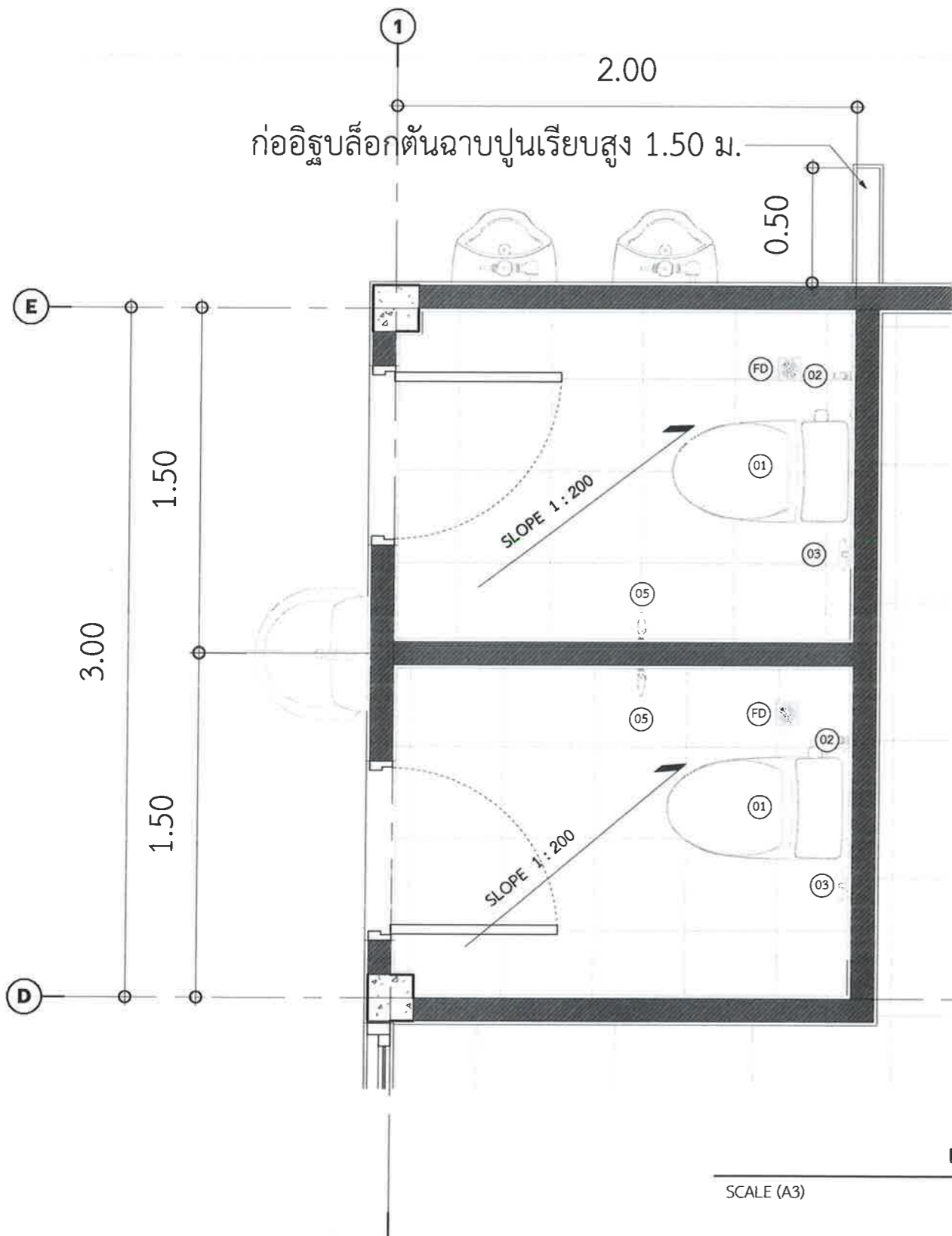
แปลนห้องน้ำ
