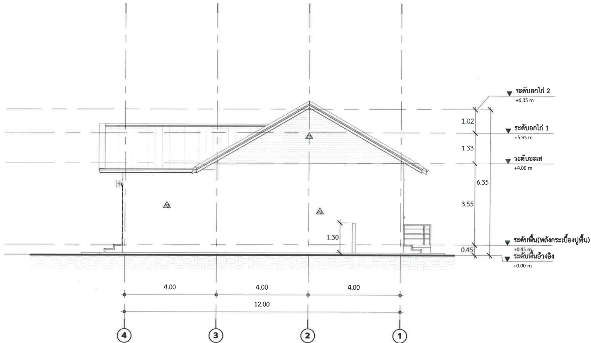
รูปด้าน 03
