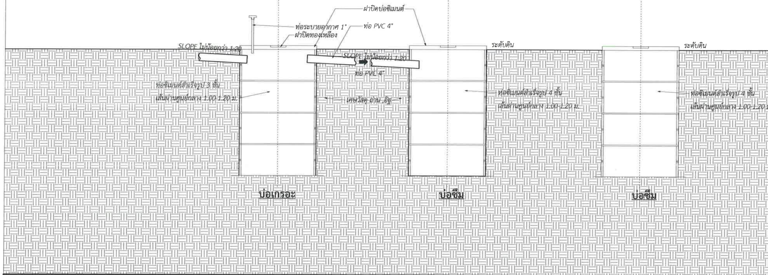
แบบขยายบ่อเกรอะ - บ่อซึม
