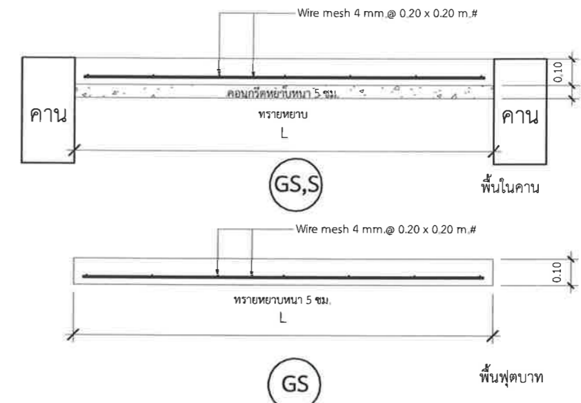
แบบขยายโครงสร้างพื้น
