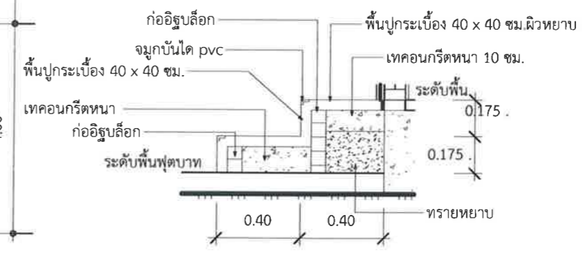
แบบขยายบันได SCALE (A3) 1 : 25
