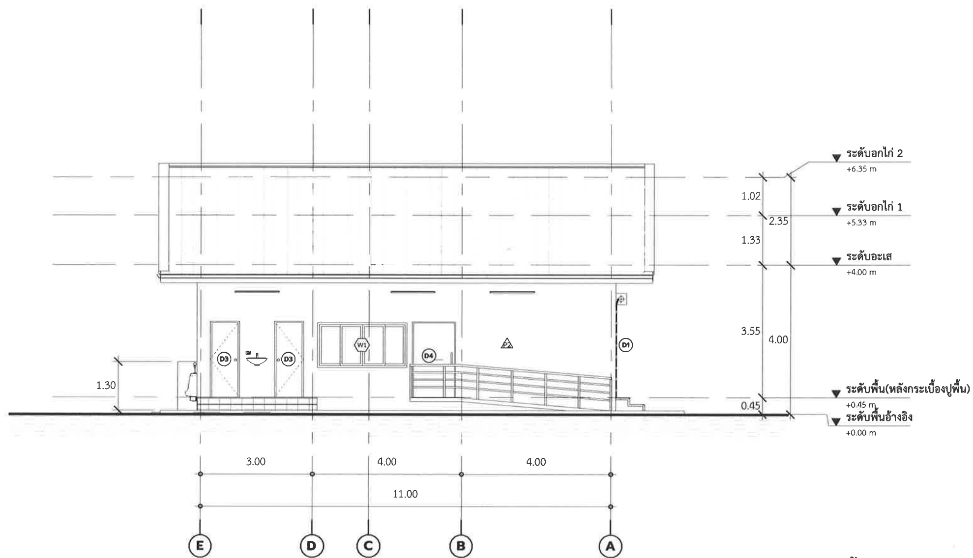
รูปด้าน 02
