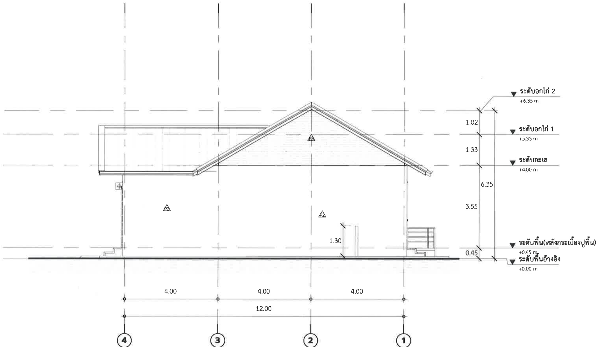
รูปด้าน 03
