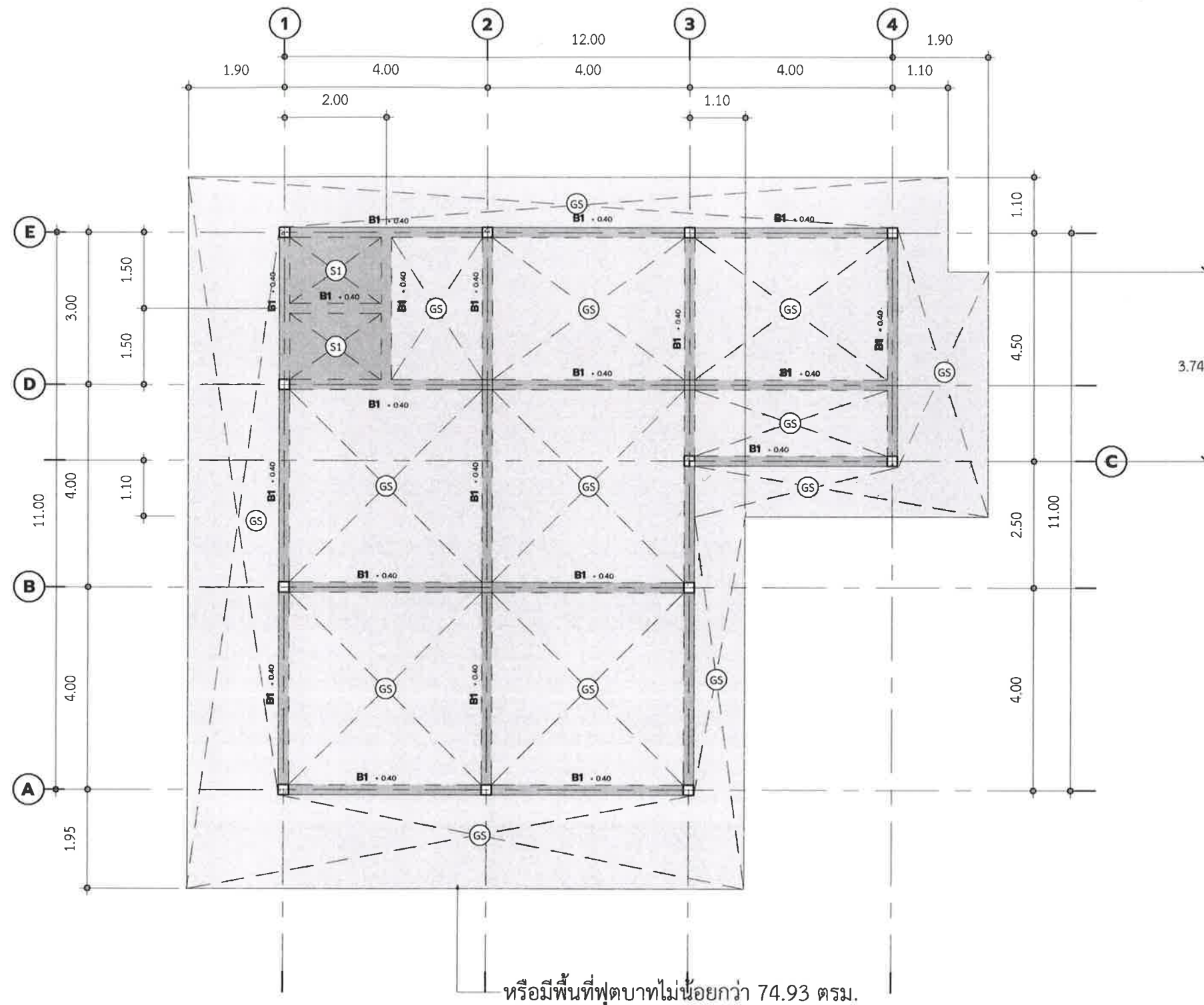
แปลนโครงสร้างคาน, พื้น ชั้นที่ 1
