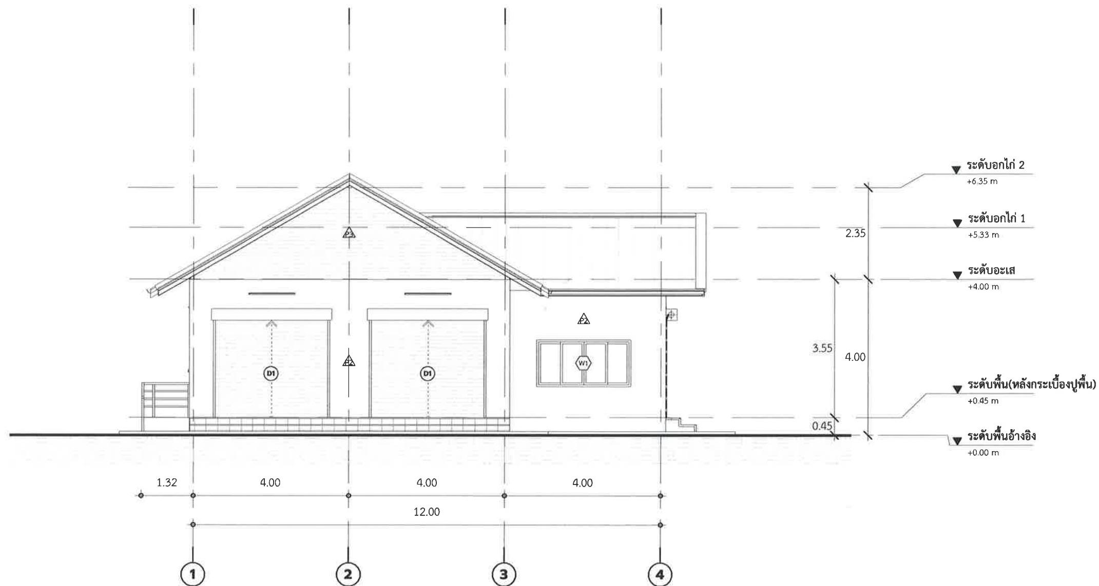
รูปด้าน 01
