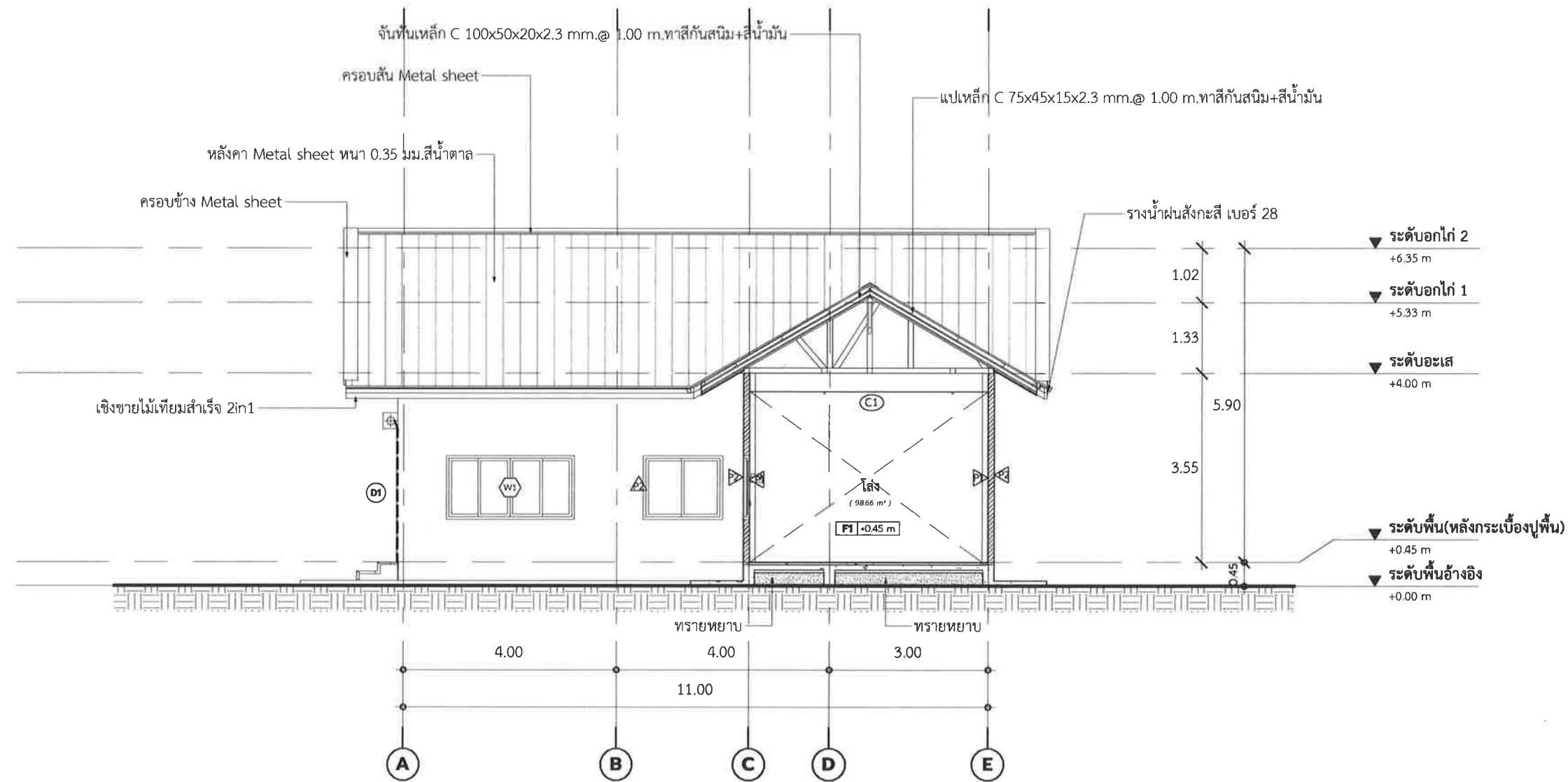
รูปตัด 02
