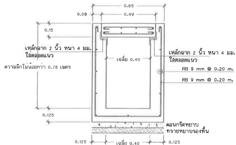
รูปตัดรางระบายน้ำ จุดที่ 1 STA 0+020 ม. Scale no
