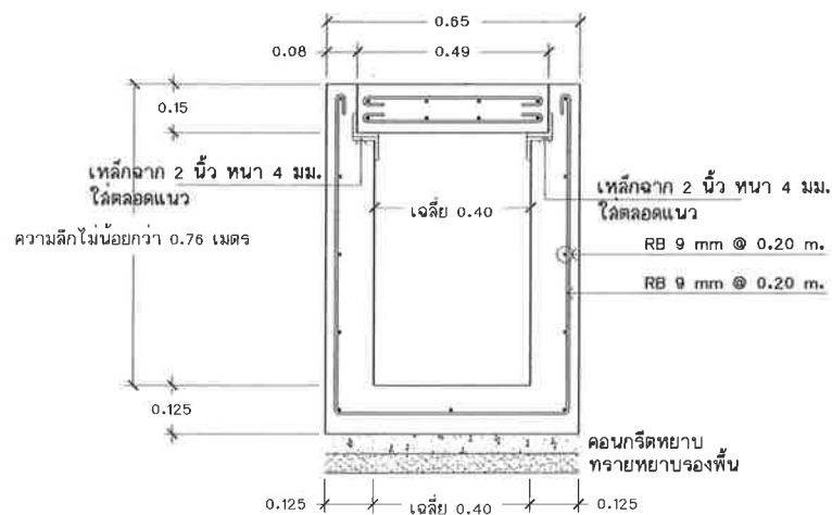
รูปตัดวางระบายน้ำ จุดที่ 1 STA 0+040 ม. Scale 1:15
