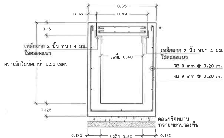
รูปตัดรางระบายน้ำ จุดที่ 1 STA 0+000 ม. Scale no
