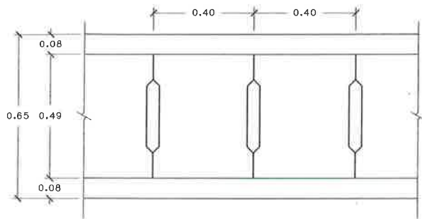
แปลนวางระบายน้ำความกว้างภายในเฉลี่ย 0.40 เมตร Scale 1:15
