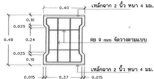
แปลนวางระบายน้ำความกว้างภายในเฉลี่ย 0.40 เมตร (หรือเฉลี่ยตามสภาพพื้นที่) Scale 1:15
