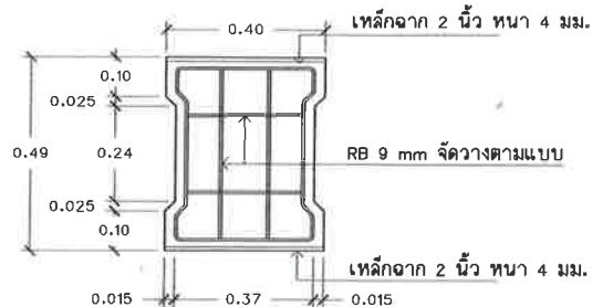
แปลนฝารางระบายน้ำความกว้างภายในเฉลี่ย 0.40 เมตร(หรือเฉลี่ยตามภาพพื้นที่) Scale 1:15
