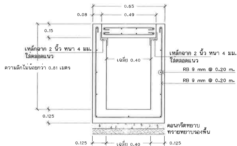
รูปตัดวางระบายน้ำ จุดที่ 1 STA 0+54 ม. Scale 1:15
