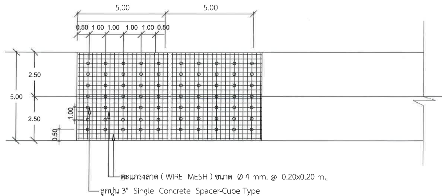
แบบการวางลูกปูน Concrete Spacer
