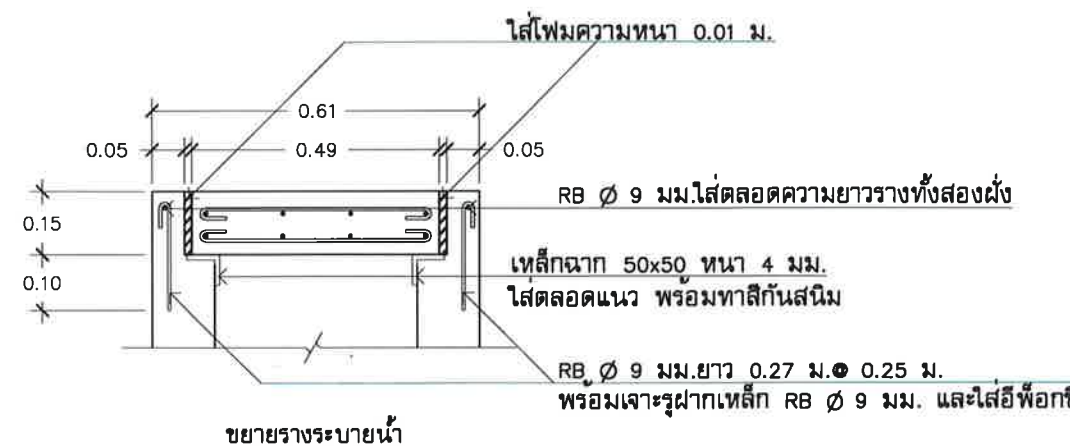
รูปตัดรางระบายน้ำ จุดที่ 1 Scale no
