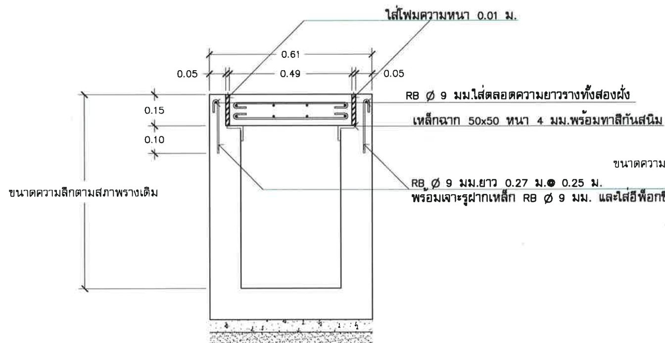
รูปตัดรางระบายน้ำ จุดที่ 1 Scale no
