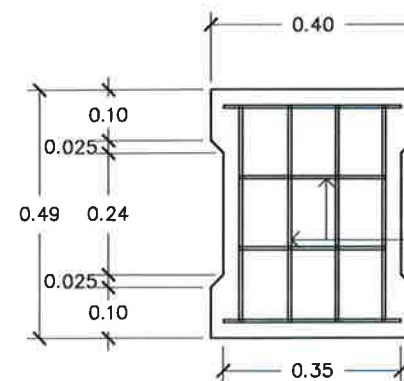
แปลนฝารางระบายน้ำความกว้างภายในเฉลี่ย 0.40 เมตร(หรือเฉลี่ยตามสภาพพื้นที่) Scale 1:15
